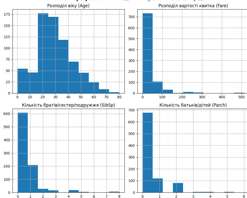
Рис. 2. Гістограми розподілу числових даних «Титанік»
